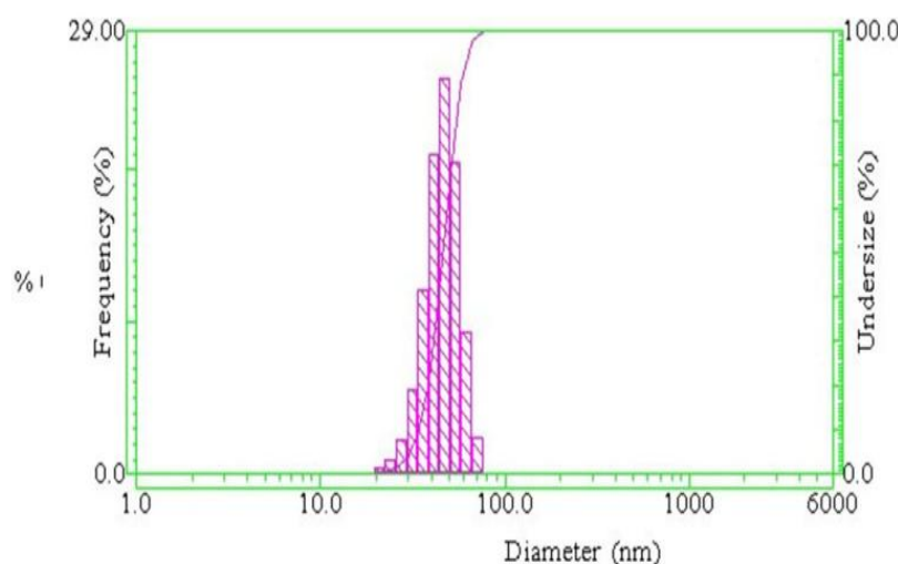
شکل ۱: نمودار توزیع اندازه نانو ذرات سنتز شده
