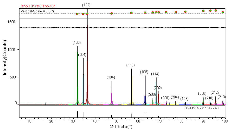
شکل ۳: نمونه الگوی پراش پرتو ایکس (XRD) از نانو ذرات اکسیدروی سنتز شده
