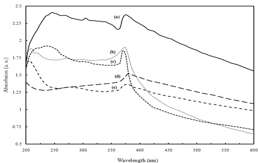
شکل ۴: طیف جذبی UV – vis برای نانو ذرات اکسیدروی سنتز شده بعد از نیم ساعت اولترا سونیک
