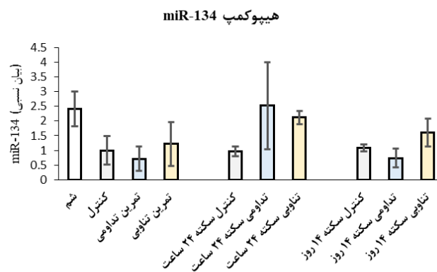
شکل ۴: تغییرات miR-134 در ناحیه هیپوکامپ، عدم تفاوت معنی دار میان گروه‌های پژوهش ( P=0/1 ).
