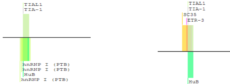
شکل ۴: آنالیز چندشکلی ژن TP53 توسط نرم‌افزار آنلاین Splice Aid2 A: عدم اتصال دو پروتئین SC35 و ETR-3؛ B: اتصال دو پروتئین SC35 و ETR-3.
