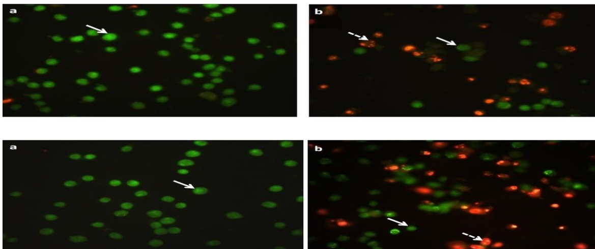
شکل ۳: نتایج مربوط به میکروسکوپ فلورسنت در رده سلولی (A) و Nalm6 (B) عصاره اتیل استاتی هسته زردآلو کنترل (A) و KG1 (B) عصاره اتیل استاتی هسته زردآلو
