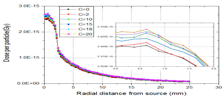
شکل ۶: دز بر حسب فاصله شعاعی تا چشمه برای غلظت‌های ۲۰، ۱۵، ۱۰، ۲، ۱۸ و ۲۰ میلی گرم نانوذرات طلا در یک گرم بافت نرم در تابش فوتون از چشمه ایریدیوم.
