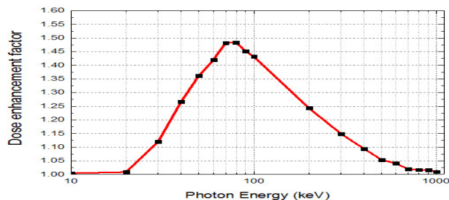
شکل ۲: تغییرات DEF بر حسب انرژی فوتون از ۱۰ keV تا ۱۰۰۰ keV در حضور نانوذر طلا با غلظت ۲۰ میلی گرم طلا در یک گرم بافت نرم.
