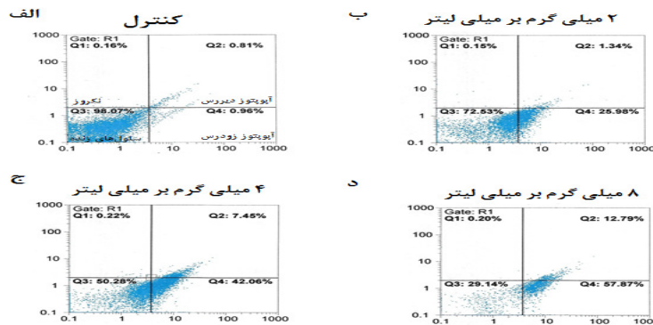
شکل ۲: منحنی تراکمی خروجی دستگاه فلوسایتومتر در اثر تیمار سلول‌های MCF-7 سرطان پستان با غلظت‌های (الف) صفر (کنترل)، (ب) غلظت ۲ میلی‌گرم بر میلی‌لیتر (ج) غلظت ۴ میلی‌گرم بر میلی‌لیتر و (د) غلظت ۸ میلی‌گرم بر میلی‌لیتر کروسین.
