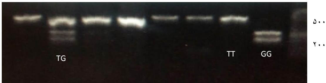
شکل ۱: نتیجه هضم آنزیمی پلی مورفیسم rs 2241766 توسط SmaI. در این شکل طول قطعات بریده شده بوسیله آنزیم نمایش داده شده است. ژنوتیپ TG سه باند با طول های ۳۷۲ bp و ۲۰۹bp و ۱۶۳bp؛ ژنوتیپ TT یک باند با طول ۳۷۲ bp
