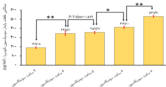
شکل ۸: تعیین میانگین غلظت پایدار سوسپانسیون نانوسریا در حضور SDS ۰/۰۵wt% با زمان های سونیکاسیون متفاوت سوسپانسیون.
