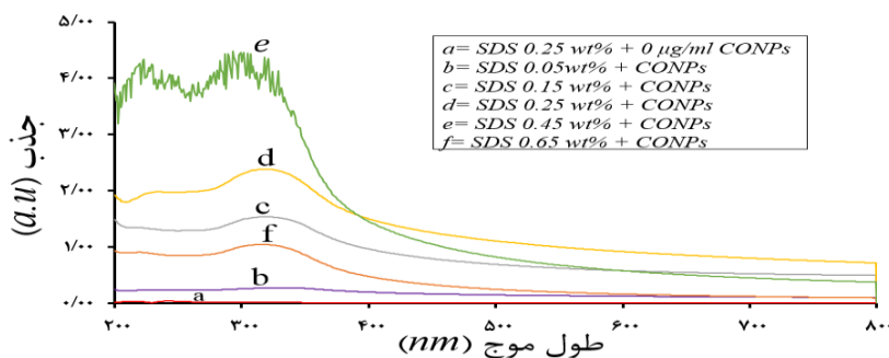
شکل ۳: طیف جذب نانوذرات سریم اکساید در حضور غلظت‌های مختلف از سورفکتانت آنیونی سدیم دودسیل سولفات (SDS)
