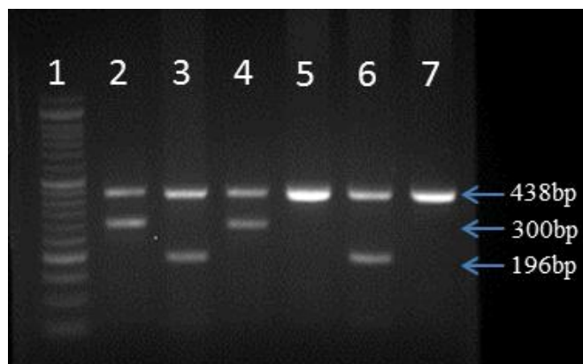
شکل ۱: نتایج حاصل از الکتروفورز محصولات ARMS-PCR بر روی ژل آگارز ۲ درصد؛ ستون ۱: نشانگر مولکولی ۵۰ جفت بازی؛ ستون ۲ و ۳ محصولات مربوط به فرد هتروزایگوت AG؛ ستون ۴ و ۵: محصولات مربوط به فرد هموزایگوت AA؛ ستون ۶ و ۷: محصولات مربوط به فرد هموزایگوت GG.
