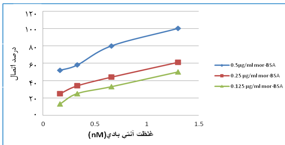
نمودار ۱: منحنی محاسبه افینیتی مربوط به آنتی‌بادی منوکلونال علیه مورفین
