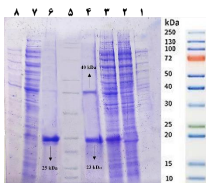
شکل ۲. الگوی الکتروفورز بیان و تخلیص آنتیژن کایمر SUMO-c-CfTXB و آنتیژن c-CfTXB در دمای ۳۷ درجه سانتی‌گراد در حضور غلظت ۱۰۰ میلی‌مولار از IPTG؛ (۱) شاهد SUMO-c-CfTXB در بافر B، (۲) بیان در SUMO-c-CfTXB در PBS، (۳) بیان SUMO-c-CfTXB در بافر B، (۴) تخلیص SUMO-c-CfTXB در بافر B با ایمیدازول ۲۰۰، (۵) نشانگر پروتئینی، (۶) تخلیص c-CfTXB در بافر B با ایمیدازول ۲۵۰، (۷) بیان c-CfTXB در بافر B، (۸) شاهد c-CfTXB در بافر B
