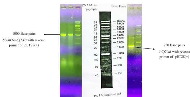
شکل ۱. الگوی الکتروفورز افقی حاصل از PCR کلونی‌های ترانسفورم شده در میزبان پروکاریوتی
