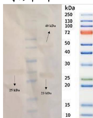
شکل ۳. تایید پروتئین نو ترکیب بیان شده به وسیله وسترن بلات با استفاده از کانژوگه موشی؛ (۱) بیان پروتئین SUMO-c-CfTXB در بافر B، (۲) نشانگر پروتئینی، (۳) بیان پروتئین c-CfTXB در بافر B
