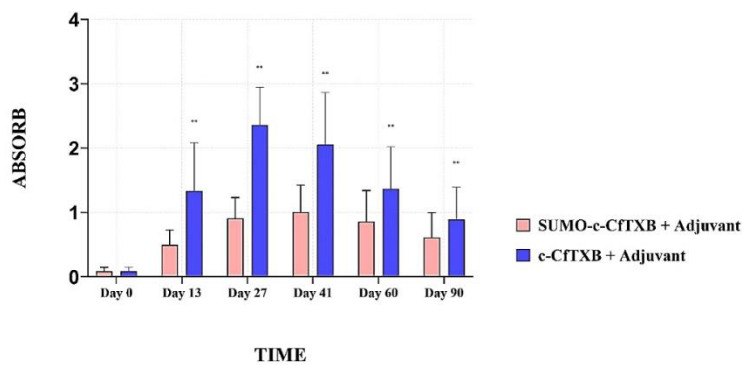
شکل ۴: نمودار آنالیز آماری جهت قیاس میزان تولید آنتی‌بادی در گروه‌های واکسینه‌شده نسبت به یکدیگر در طول موج ۴۹۰ نانومتر
