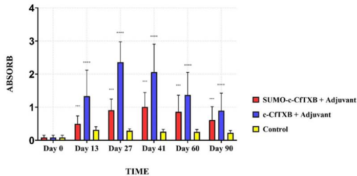
شکل ۳: نمودار آنالیز آماری مربوط به تولید آنتی‌بادی در گروه‌های واکسینه‌شده نسبت به کنترل منفی در طول موج ۴۹۰ نانومتر
