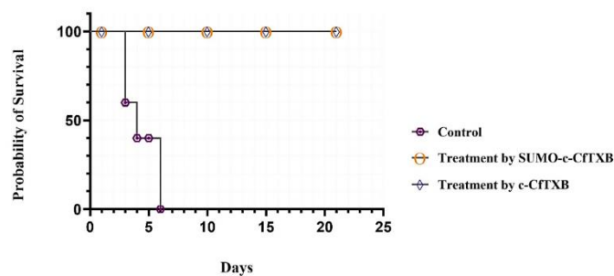
شکل ۶: نمودار آنالیز زنده‌مانی (بقاء) گروه‌های چالش شده با توکسین عروس دریایی
