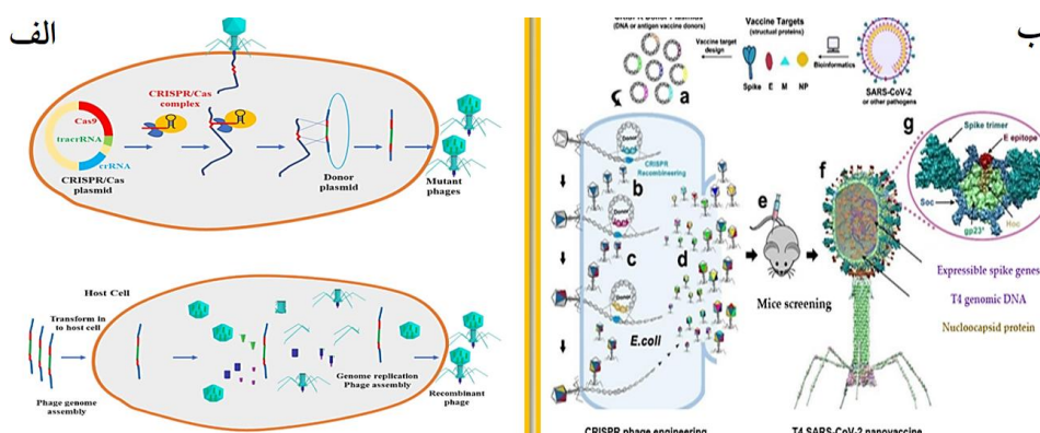
شکل ۵: الف- راه اندازی مجدد فاز و مونتاژ توسط DNA ژنومی، DNA سازواره سلول میزبان فاز با فازهای عفونی نو ترکیب جدید ترکیب می شود (۱۸). ب- مراحل ساخت نانوکاسن T4-SARS-CoV-2 با استفاده از کریسپر (۱۱).
