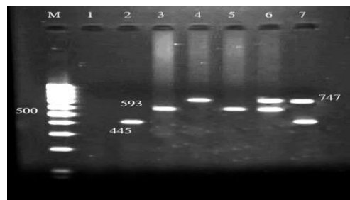
شکل ۱: ژل الکتروفورز محصول PCR ژن‌های bla CTX-M ، bla TEM و bla SHV در ایزوله‌های انتروباکتر آئروژنز. ستون M: مارکر ۱۰۰ جفت بازی فرمتاز، ستون ۱: کنترل منفی، ستون‌های ۲ و ۵: نمونه واجد ژن bla TEM ، ستون ۳: نمونه واجد ژن bla CTX-M ، ستون ۴: نمونه واجد ژن bla SHV ، ستون ۶: نمونه واجد ژن‌های bla SHV و bla CTX-M ، ستون ۷: نمونه واجد ژن‌های bla SHV و bla TEM
