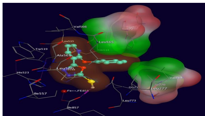
شکل ۱: بهترین نحوه اتصال پیش بینی شده در مطالعه داکینگ مربوط به ترکیب 7a به اکتیو سایت آنزیم لیپواکسیژناز (رنگ سبز نشان دهنده نواحی هیدروفوب و رنگ قرمز نواحی هیدروفیل را نشان می دهد. جهت وضوح بهتر لیگاند به صورت گوی و میله ترسیم شده است. پیوند هیدروژی به رنگ صورتی مشخص شده است)
