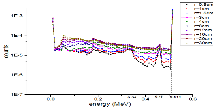
شکل ۴: تابع پاسخ آشکارساز برای چشمه حجمی کروی یکنواخت با شعاع‌های مختلف در داخل کره ای از بافت نرم به همان شعاع
