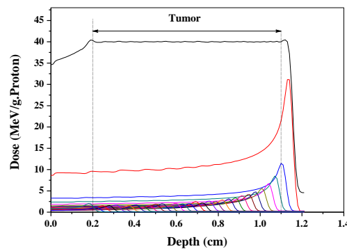
نمودار ۳: قله براگ پهن شده (SOBP) ایجاد شده از باریکه پروتون ۳۲/۸۵ MeV و چرخ مدولاتور
