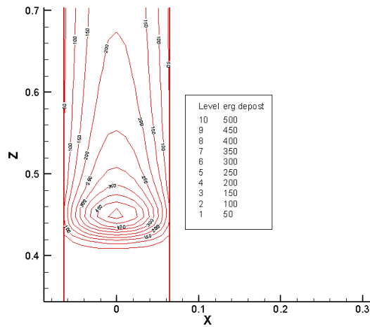
نمودار ۵: نمودارهای هم‌دوز برای پروتون‌های با انرژی ۳۲/۸۵ MeV
