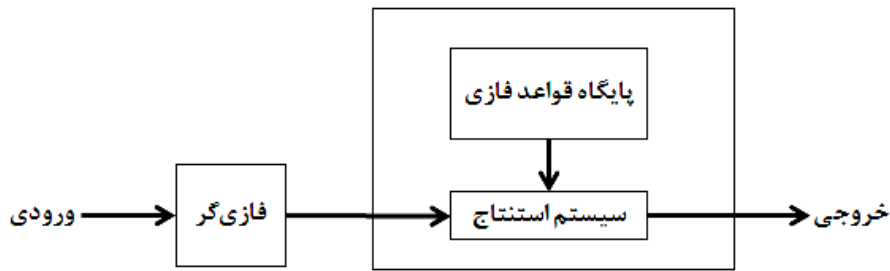
شکل ۱: بلوک دیاگرام سیستم فازی تاگاکای-سوگنو
