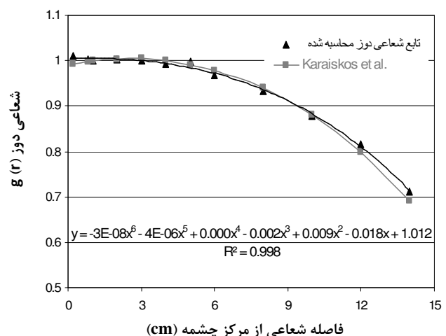
نمودار ۲: تابع شعاعی دوز، g(r) ، برای چشمه ایریدیم-۱۹۲
