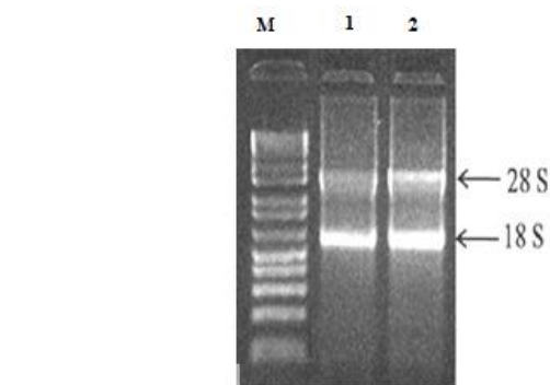
شکل ۳: نتایج استخراج RNA روی ژل آگارز ۱ درصد 50 bp Ladder (M)
