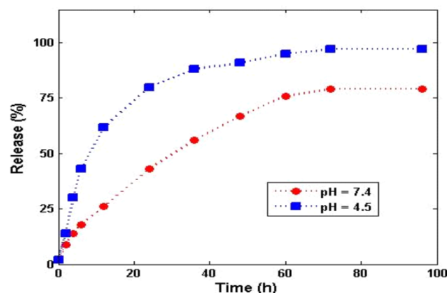
شکل ۵: نمودار رهایش کارکامین از نانوکامپوزیت در دو بافر مختلف (pH ۷/۴ و pH ۴/۵) در pH ۴/۵ میزان رهایش نسبت به pH ۷/۴ بالاتر است
