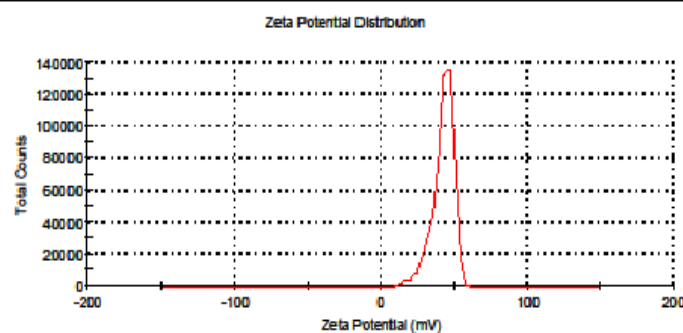
شکل ۴: پتانسیل زتای به دست آمده از نانوکامپوزیت پلی ساکاریدی کیتوزان- نشاسته- مونت موریلونیت بارگذاری شده با کارکامین
