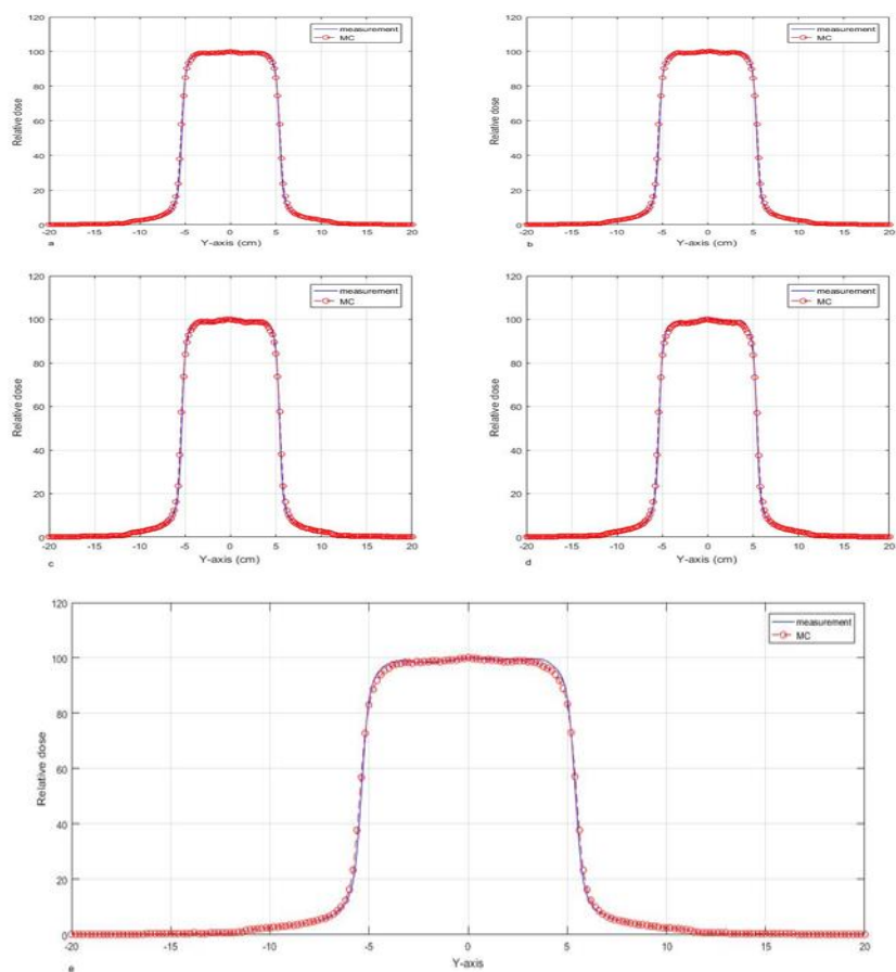
شکل ۵: منحنی های پروفایل دز برای دسته پرتو با انرژی ۱۸ مگا ولتاژ و اندازه میدان ۱۰ در ۱۰ و FWHM = 0.12 (a) انرژی ۱۴ مگا الکترون ولت، (b) ۱۴/۲ مگا الکترون ولت، (c) ۱۴/۴ مگا الکترون ولت، (d) ۱۴/۶ مگا الکترون ولت و (e) ۱۴/۸ مگا الکترون ولت
