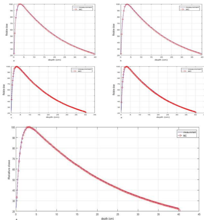
شکل ۳: منحنی های درصد دز عمقی برای دسته پرتوهای با انرژی ۱۸ مگا ولتاژ و اندازه میدان ۱۰×۱۰ (a) انرژی ۱۴ مگا الکترون ولت (b) انرژی ۱۴/۲، (c) انرژی ۱۴/۴ مگا الکترون ولت، (d) انرژی ۱۴/۶ مگا الکترون ولت و (e) انرژی ۱۴/۸ مگا الکترون ولت
