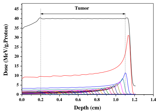
نمودار ۳: قله براگ پهن شده (SOBP) ایجاد شده از باریکه پروتون 32/85 \text{ MeV} و چرخ مدولاتور
