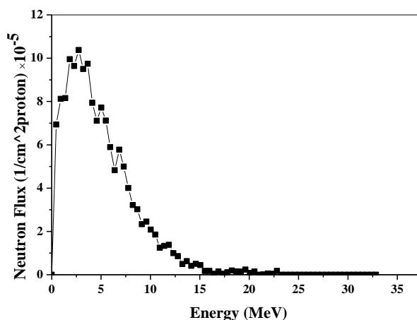
نمودار ۹: طیف انرژی نوترون‌ها در تومور
