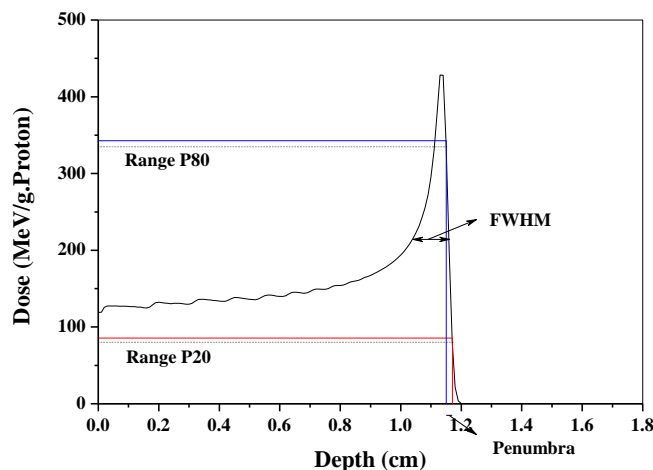
نمودار ۲: منحنی براگ باریکه پروتون با انرژی ۳۲/۸۵ MeV
