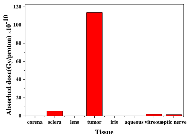
نمودار ۸: دوز دریافتی کل (مجموع دوز پروتون‌ها و ذرات ثانويه) در بافت‌های چشم
