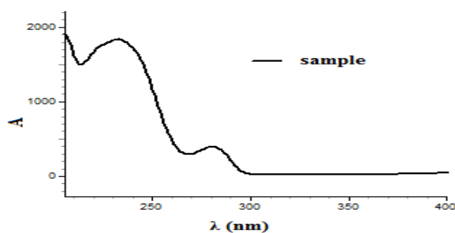
شکل ۴: طیف اسپکتروفتومتری نمونه اولئوروپین استخراج شده در ناحیه ۰ تا ۴۰۰ نانومتر حداکثر جذب اولئوروپین در طول موج ۲۳۰ نانومتر و ۲۷۰ نانومتر
