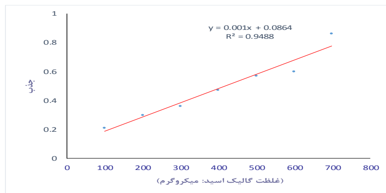
نمودار ۱: منحنی استاندارد گالیک اسید با دستگاه اسپکتروفتومتر
