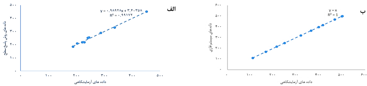
شکل ۲: نمودار مقادیر پیش‌بینی شده بر حسب مقادیر آزمایشگاهی فرآیند الکتروپرسی.
