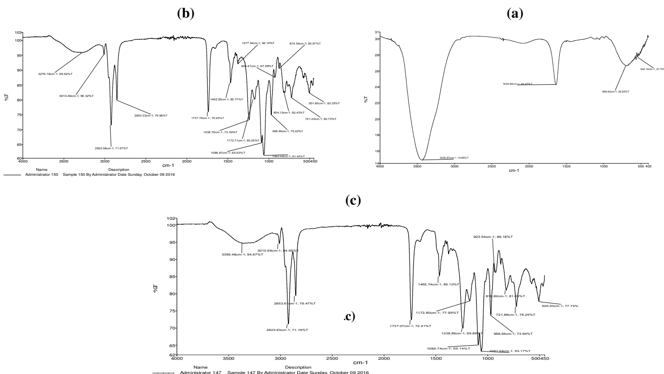
تصویر ۱: (a) آنالیز FTIR عصاره خالص آناناس، (b) آنالیز FTIR سامانه لیپوزومی خالی (بلانک)، (c) آنالیز FTIR نانولیپوزوم حاوی عصاره آناناس
