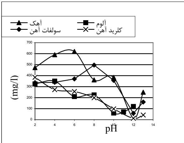
نمودار ۱: بهینه PH برای مواد منعقد کننده استفاده شده
