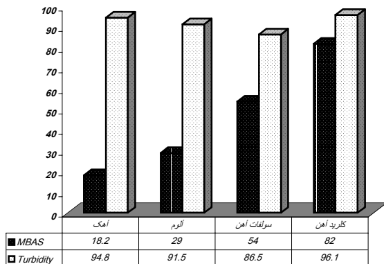
نمودار ۳: تأثیر مواد منعقد کننده بر حذف کدورت و مواد فعال سطحی
